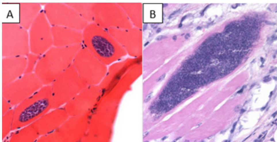
Figuur 2: Sarcocyste(n) van Sarcocystis spp. ingebed in spierweefsel in HE (A) kleuring en in vergroting 500x (B) uit (CDC - DPDx - Sarcocystosis, n.d.).
