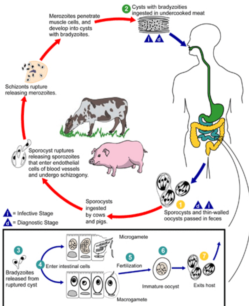
Figuur 1: Levenscyclus S. hominis en S. suis van (CDC - DPDx - Sarcocystosis, n.d.; Prevention, 2019)
