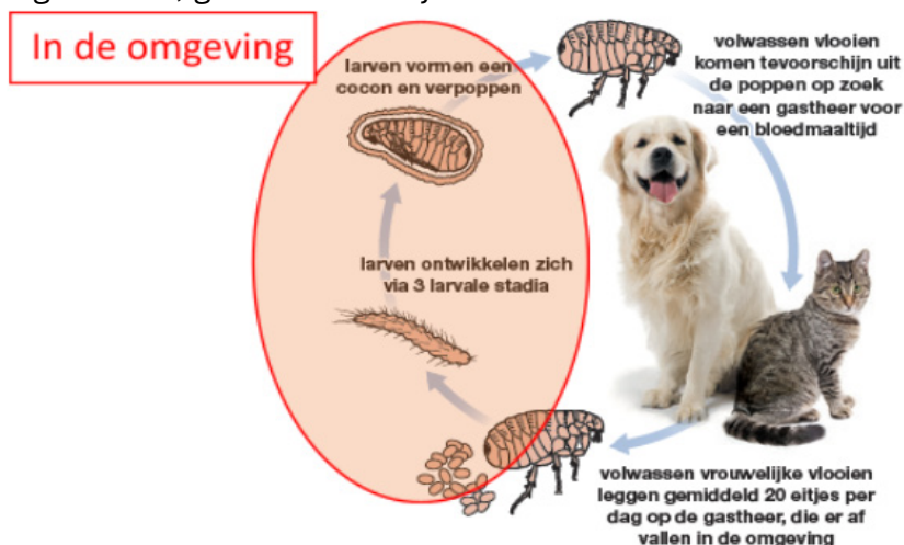
Figuur 1: Vlooienlevenscyclus Bron: Esccap 2
